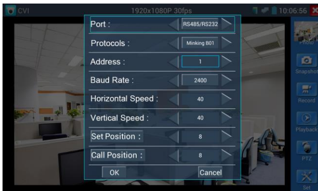
Рис.3.3.6.-4 Настройки RS-485 (2)
