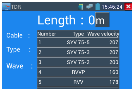
Рис. 3.3.22-2 Выбор параметров кабеля
